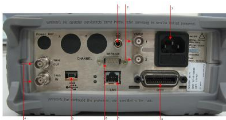
Рисунок 7 – Вид блока измерительного E4417A сзади
